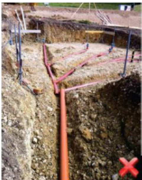
Canalisations SANS assise bétonné !
